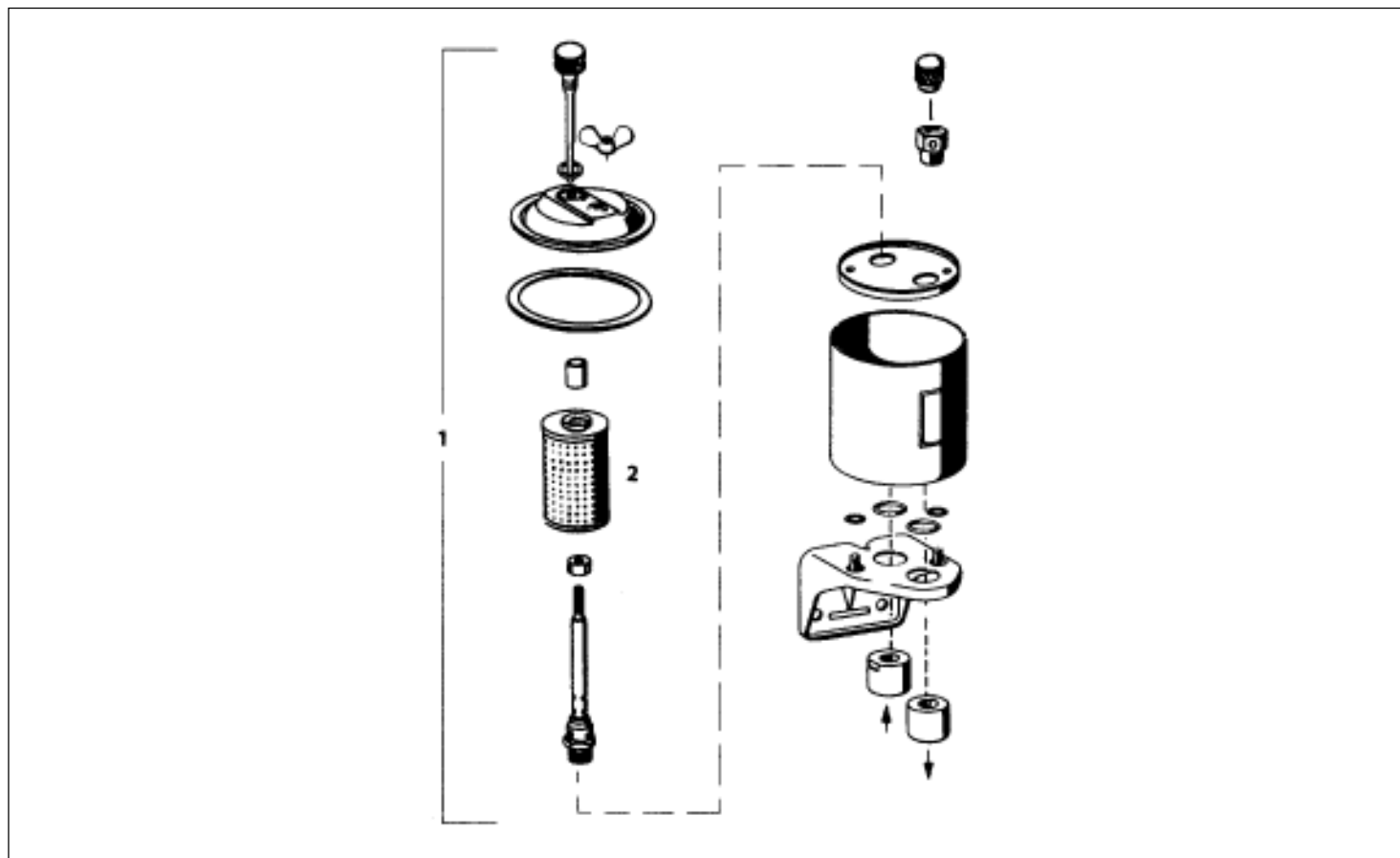
HYDRAULIC TANK (ZF)
